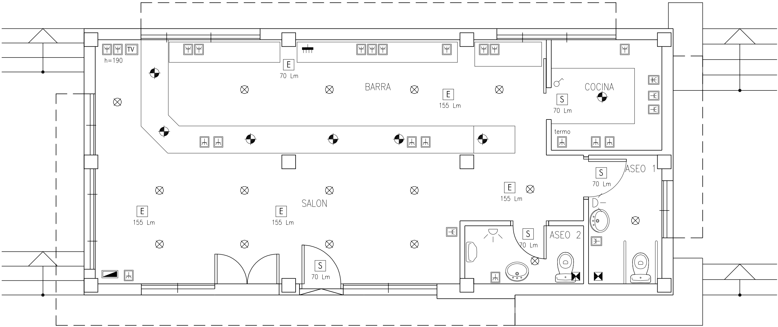
ESTADO REFORMADO : ALUMBRADO, FUERZA Y EMERGENCIA
