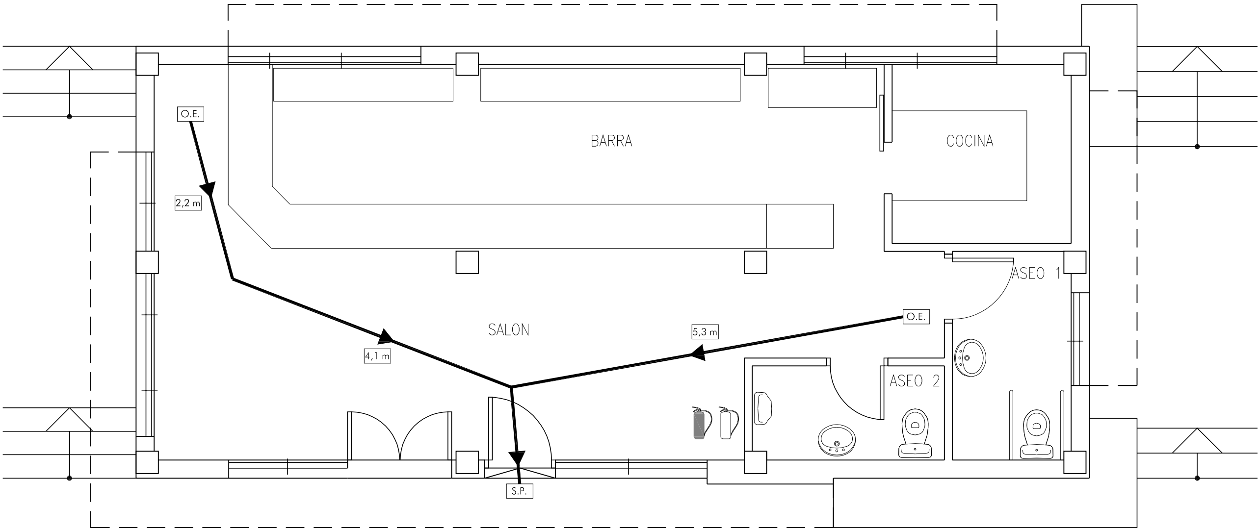
ESTADO REFORMADO : EVACUACION Y CONTRAINCENDIOS
