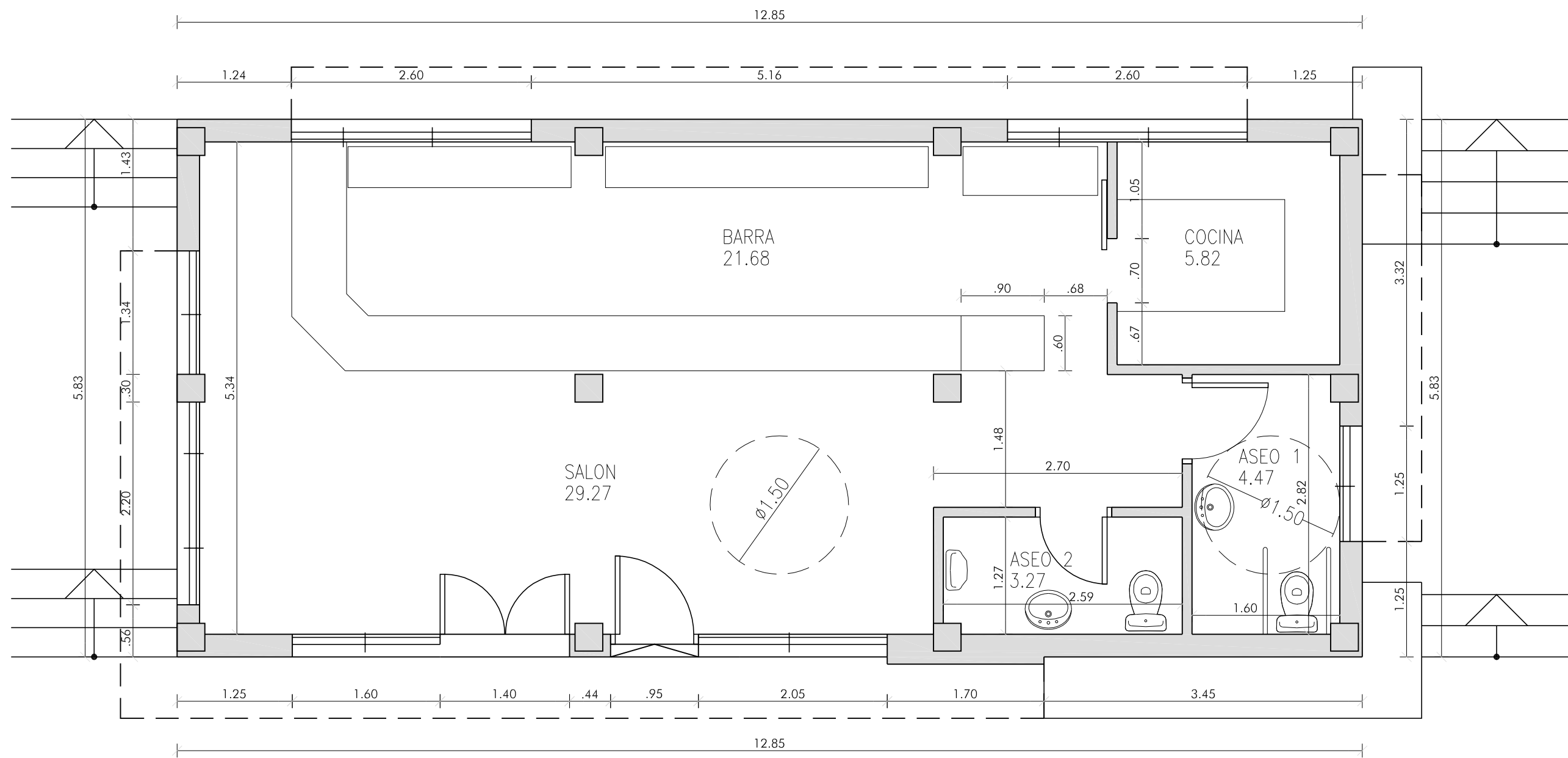
ESTADO REFORMADO : DISTRIBUCIÓN
