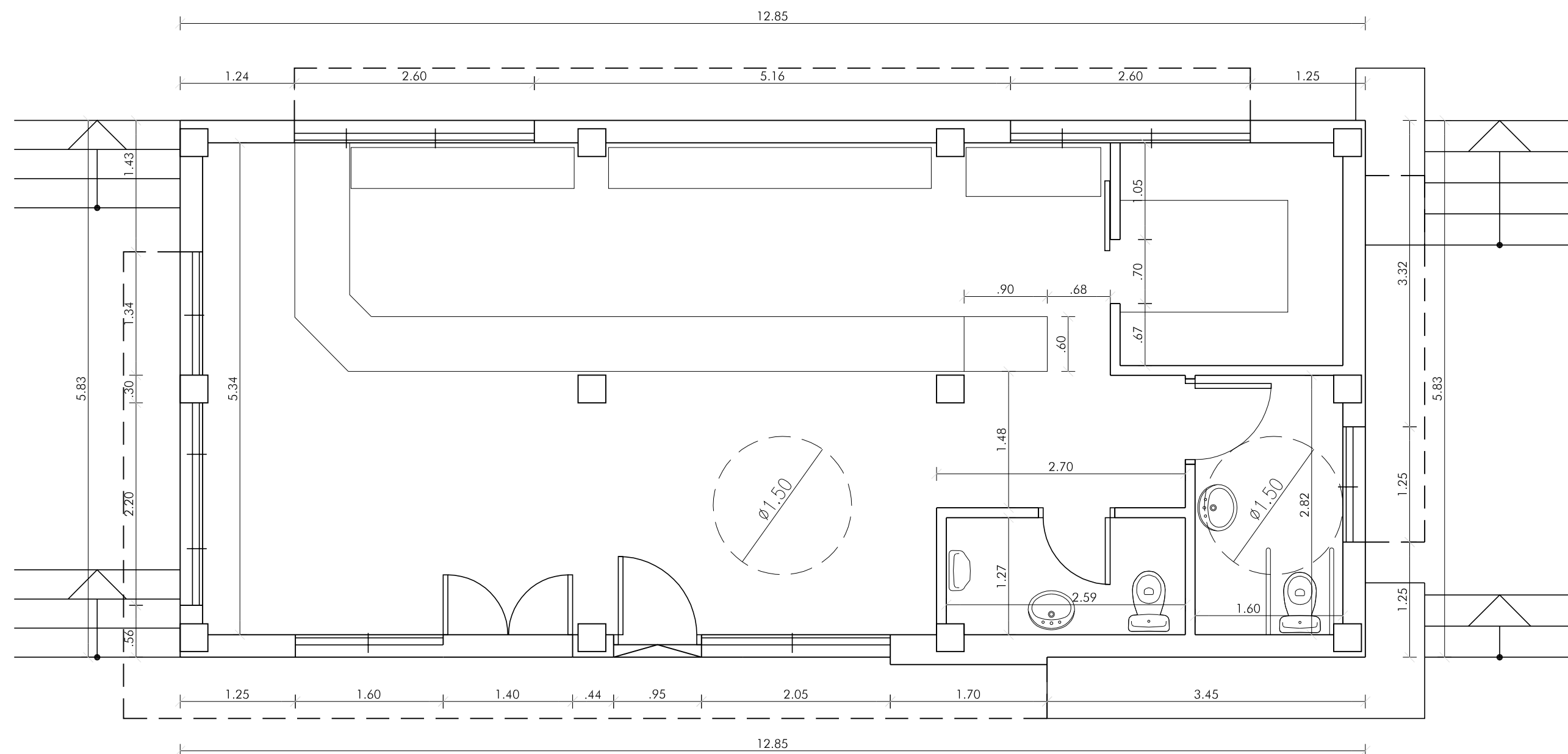
ESTADO REFORMADO : COTAS
