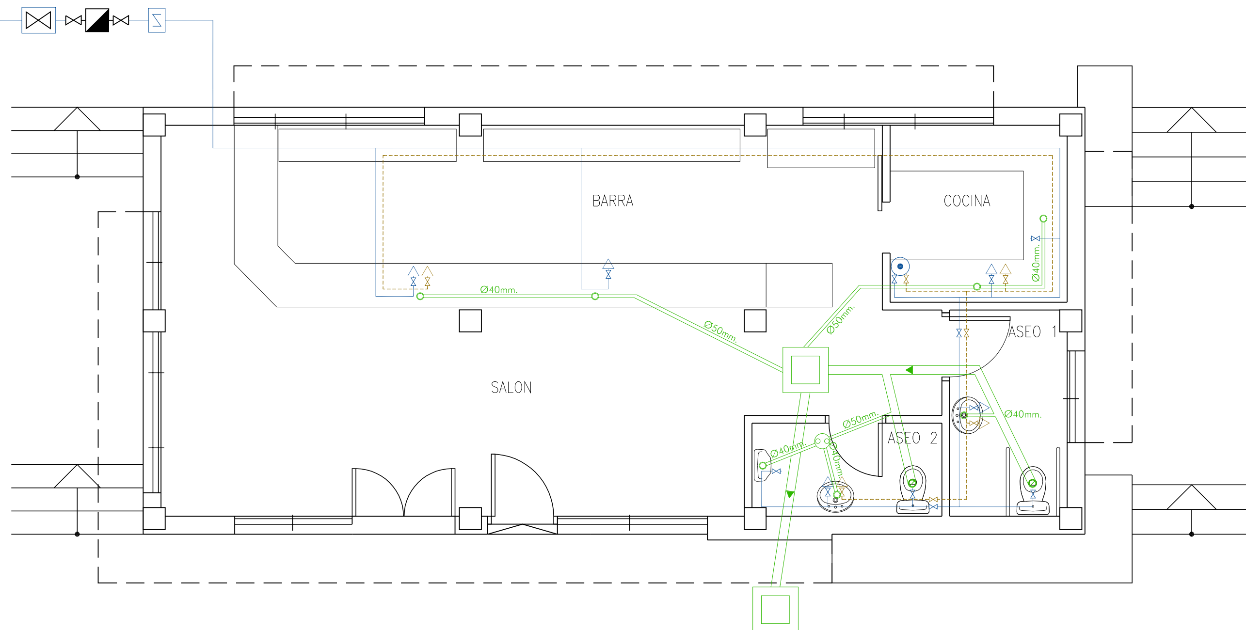
ESTADO REFORMADO : FONTANERIA Y SANEAMIENTO
