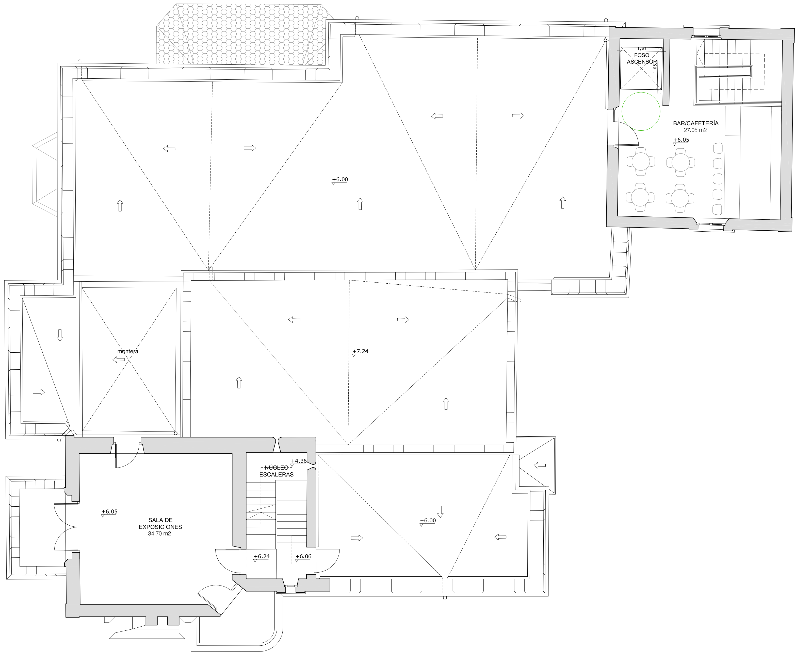
PLANTA PRIMERA
