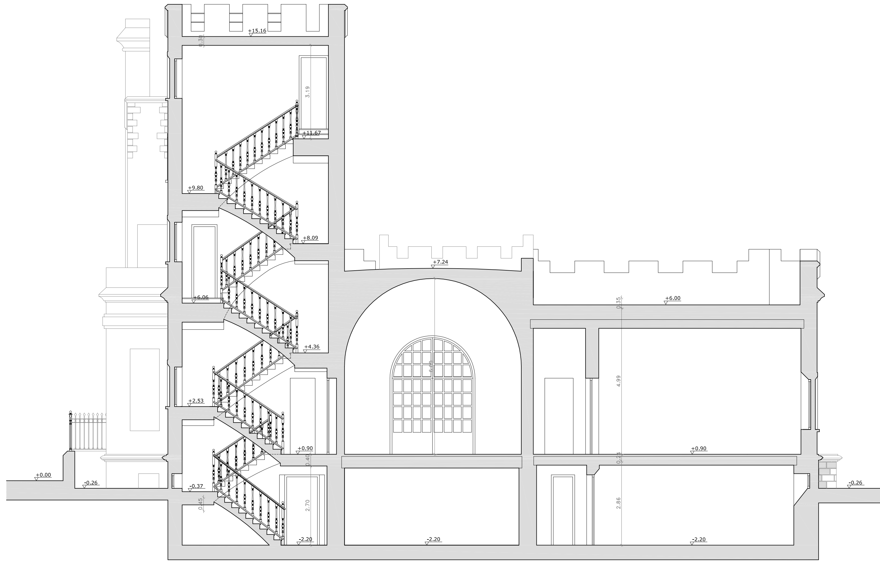
SECCIÓN 1-1
