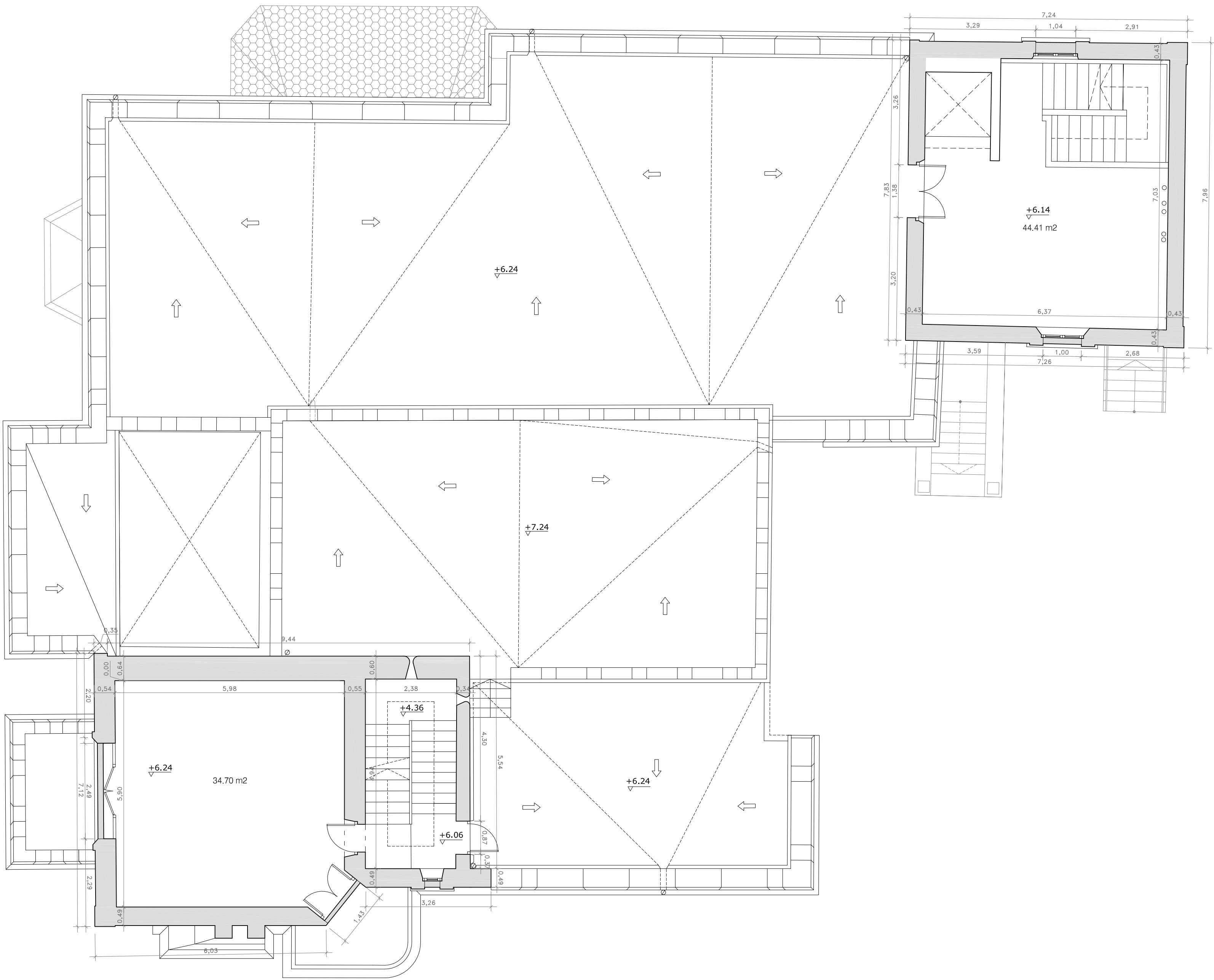
PLANTA PRIMERA
