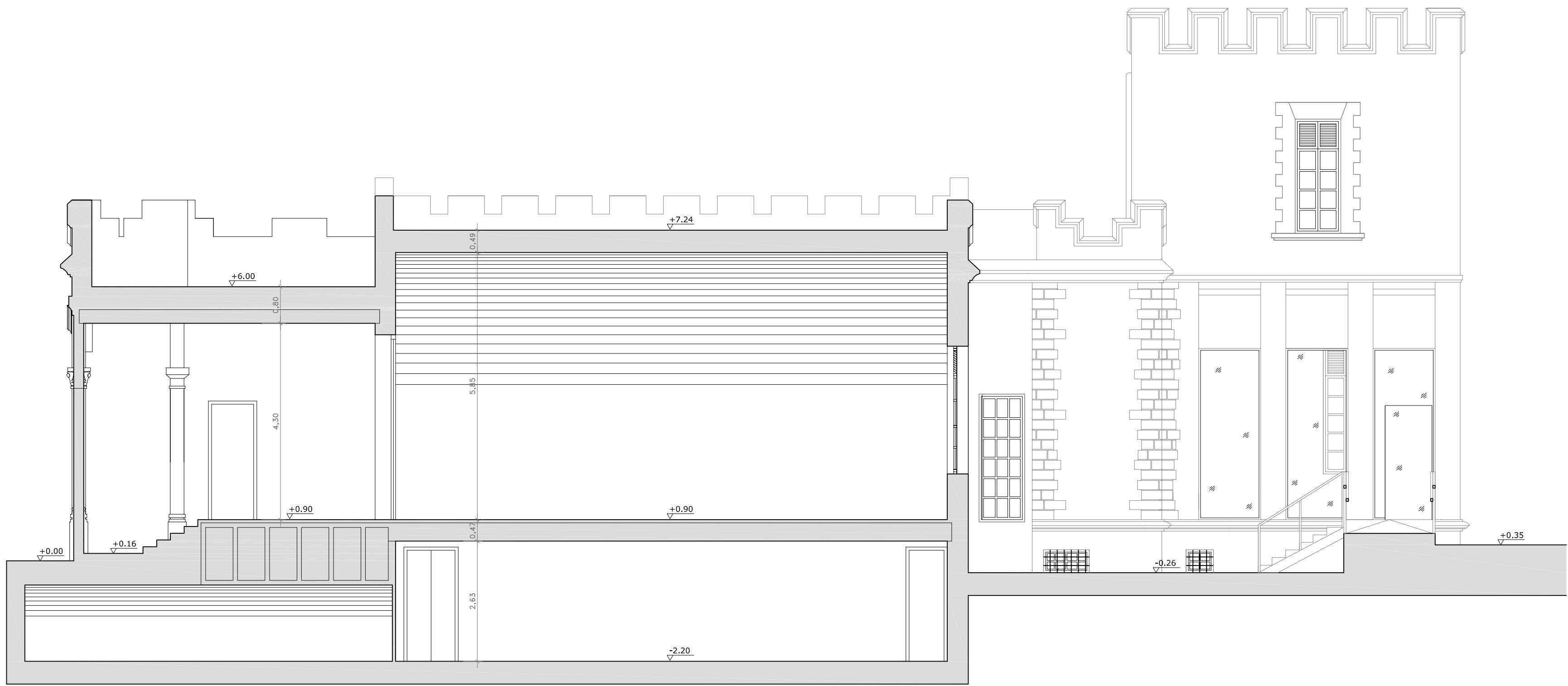
SECCIÓN 2-2
